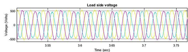
Fig.5.3. Load side voltage (SAPF)
