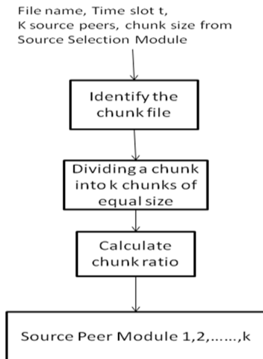
Fig.6. Data Provider Module
