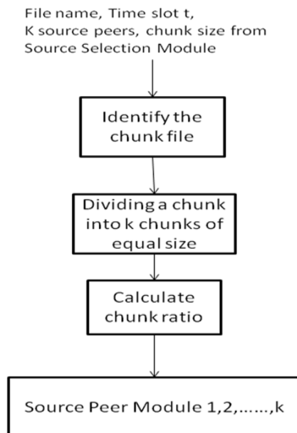
Fig. 11. Data Provider Module
