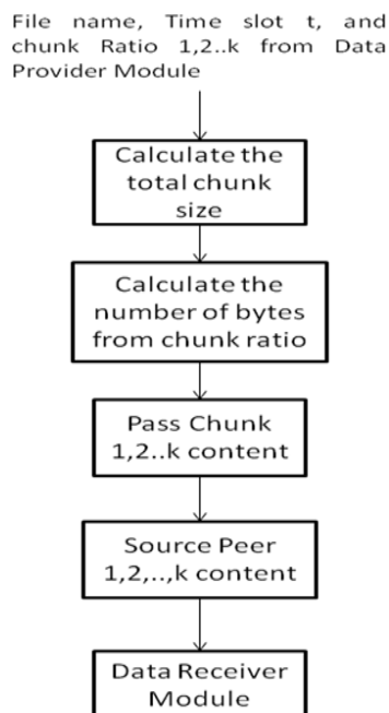
Fig.7. Source Peer Module
