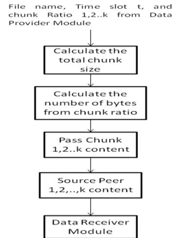
Fig.12. Source Peer Module
